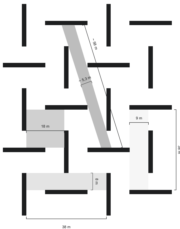
Figuur 7. Een hagelslagpatroon (variant 1, L=20\text{ m} , D=20\text{ m} , l=20\text{ m} , B=2\text{ m} en C=10\% ). De maximale ongedekte rechthoek is 18 \times 18\text{ m} ( =324\text{ m}^2 ). De maximale ongedekte ruimte in de lengterichting is 38 \times 9\text{ m} ( =342\text{ m}^2 ), loodrecht op de lengterichting 38 \times 8\text{ m} ( =304\text{ m}^2 ). In diagonale richting zijn er vier ongedekte ruimtes van circa 58 \times 5,3\text{ m} (ca. 307\text{ m}^2 ).
