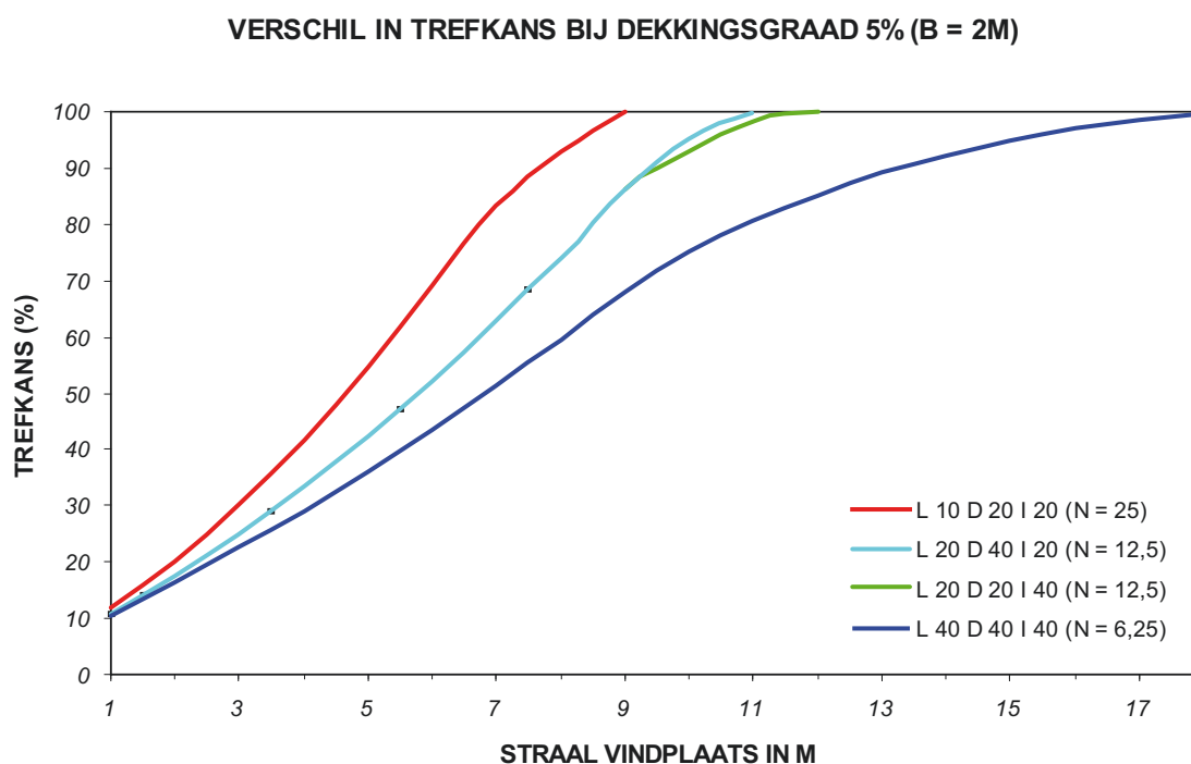
Figuur 4. Illustratie van de verschillen in trefkans bij verschillende stippelijnpatronen met gelijke dekkingsgraad. B = sleufbreedte, L = sleuflengte, D = sleufafstand, I = interval, N = aantal sleuven per hectare. Zie ook hierna.
